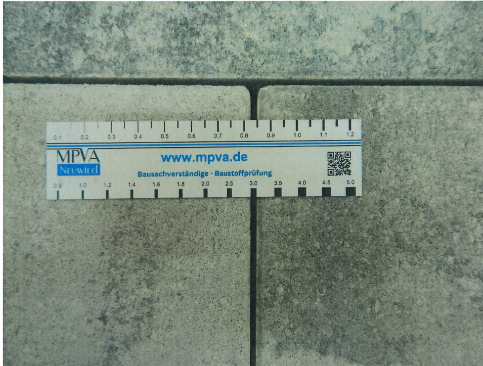
Bild 3: Resultierende Fugenbreite mit Fugenfüllung
